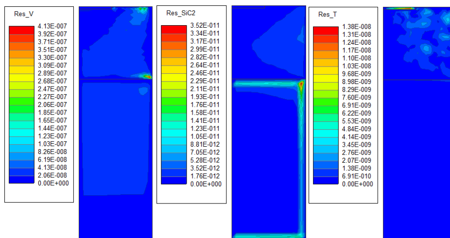
図 5. 成長層内の流速（左図）、化学種（中図）、温度（右図）の残差分布
