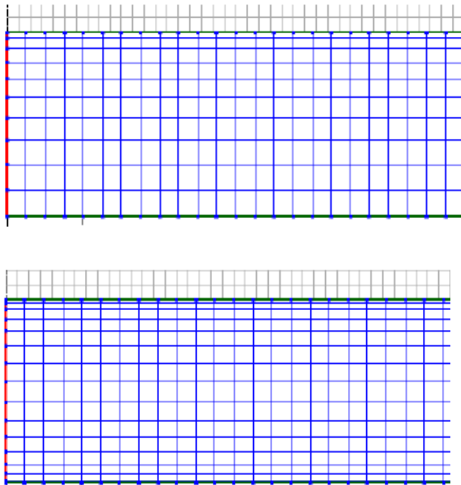
図 3. 上部にノード点を寄せた場合の計算格子（上図）、上下に寄せた場合の計算格子（下図）
