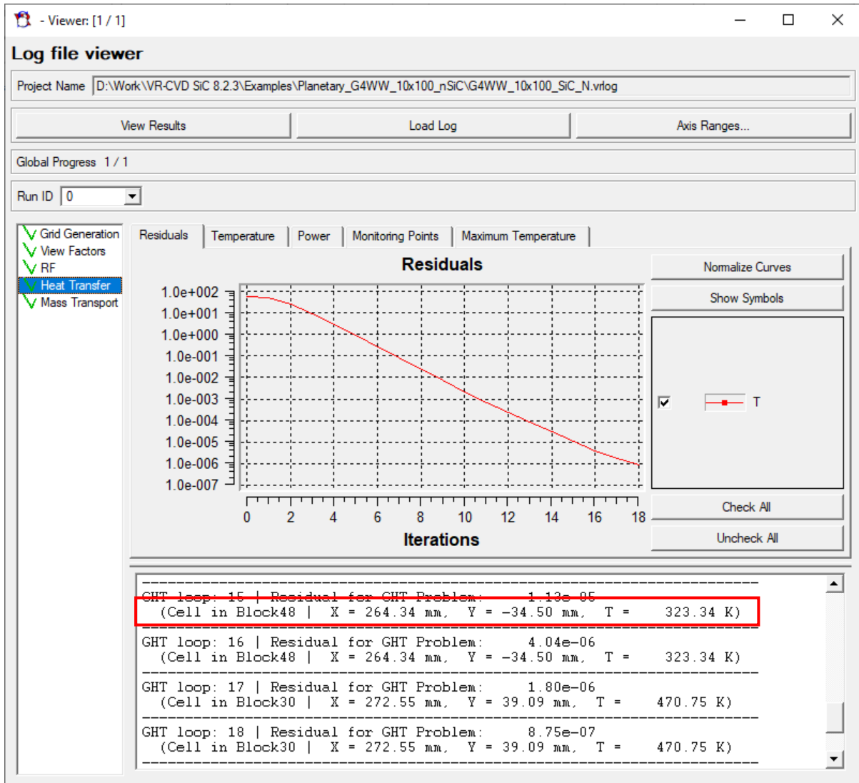
図 : Solver 画面
